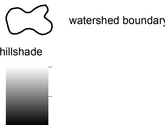
Hillshade Map
