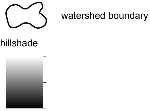
Hillshade Map
